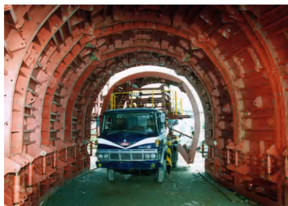
同上(型枠内部)
